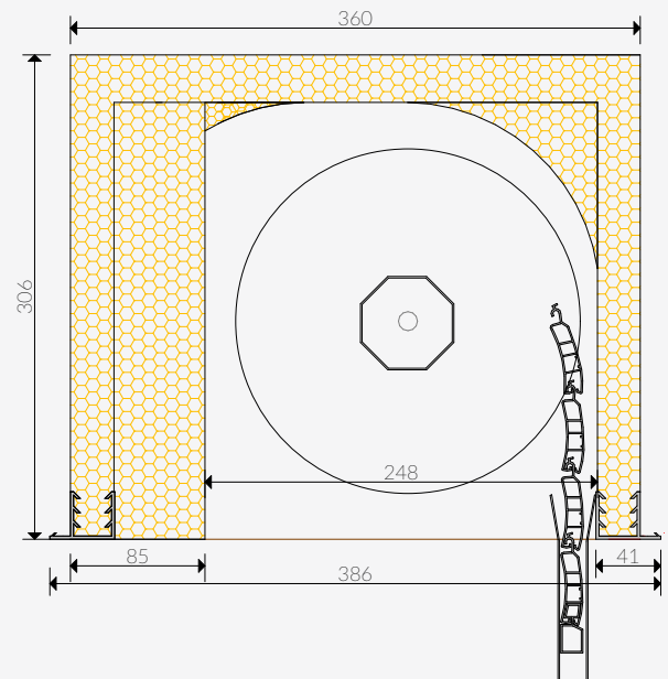
CASSONETTO TERMOTOP CS 36 TTP
