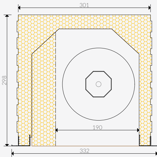
CASSONETTO TERMOPLUS CS30 TPL
